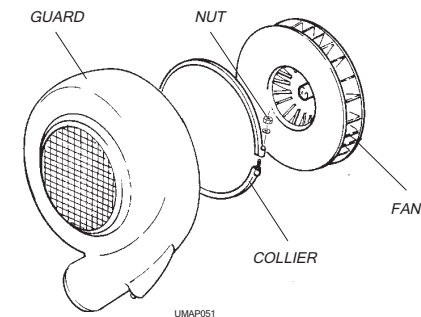
UMAP051
