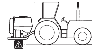
UMAP013
