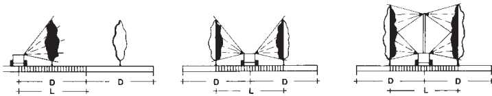
UMAP082
