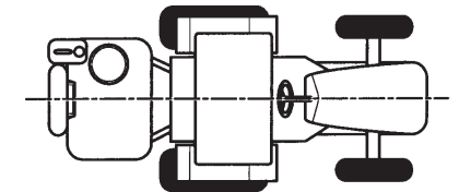
UMAP015
