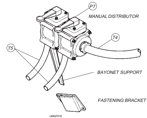
UMAP018
